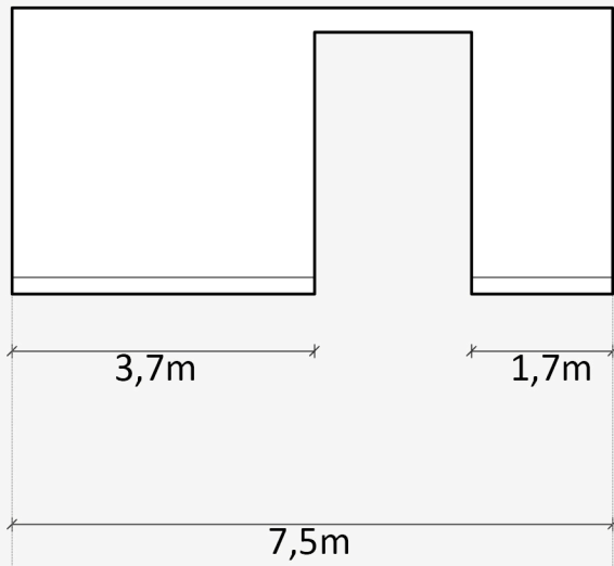
Elevación ESTE
