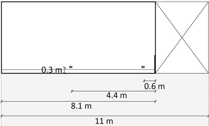
Elevación SUR
