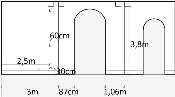
Elevación OESTE
